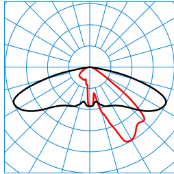
Publisca P1-AB2L-LR/5600-740 6G1S ET (CLO end value) TX301111 ■ C0 - C180 ■ C90 - C270 DIN 5040: A30 UTE: 1,00 G CEN Flux Code: 35 74 97 100 100
