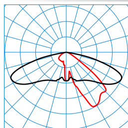
Publisca P2-AB2L-LR/4200-730 6G1S TX047761 DIN 5040: A30 UTE: 1,00 G CEN Flux Code: 35 74 97 100 100
