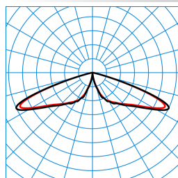
CS 19 100-RB6L-LR/5100-740 4G1S ET (CLO end value) TX300127
