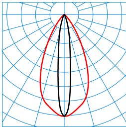
Altigo G2 C 60 SE6L/800-830 1G1P + G2 VE IP66 24V DC 80W TX113923 UGR I = 14,5 UGR q = 6,1 DIN 5040: A70 UTE: 1,00 A CEN Flux Code: 93 98 99 100 100 ■ C0 - C180 ■ C90 - C270
