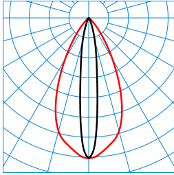
Altigo G2 C 60 SE6L/800-830 1G1P + G2 VE IP66 24V DC 240W TX113931 UGR I = 14,5 UGR q = 6,1 DIN 5040: A70 UTE: 1,00 A CEN Flux Code: 93 98 99 100 100 ■ C0 - C180 ■ C90 - C270
