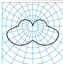
PolaroniQ WD1 LED1000-830 ETDD TX040711
