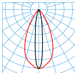
Altigo G2 10 SE6L/300-830 1G1P + G2 VE IP66 24V DC 120W TX113660
