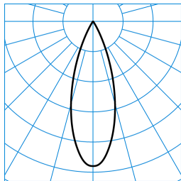
E-Line 7651 Lentyp L-FL 30-EW M48 ET 03 (225) TX463142
