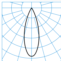
E-Line 7651 LentyP L-FL 30-EW M48 ET 03 (150) TX463141
