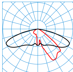
Publisca P2-AB2L-LRA/5100-730 6G1S ET (CLO end value) TX301793 DIN 5040: A30 UTE: 1,00 G CEN Flux Code: 35 74 97 100 100
