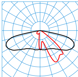
Publisca P2-AB2L/1500-740 2G1S TX047703
