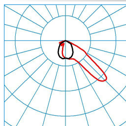
Jovie 50-AM2L-6-51-740-CLO-B
