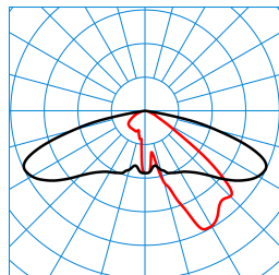
Publisca P2-AB2L-LR/5600-740 6G1S ET (CLO end value) TX300700 ■ C0 - C180 ■ C90 - C270 DIN 5040: A30 UTE: 1,00 G CEN Flux Code: 35 74 97 100 100
