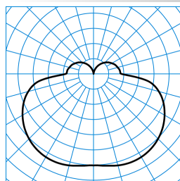
PolaronIQ WD2D LED2000-830 ET EB3 TX044282
