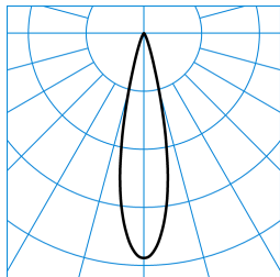
E-Line 7651 Lentyp L-SP 30-BC M49 ET 05 (225) TX463496
