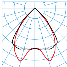
SFlow C2-L MRX LED4000-840 01 TX051991
