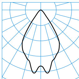
InperlaLP C05 BR22 2700-830 03 + RD-PC TX041567 ■ C0 - C180
