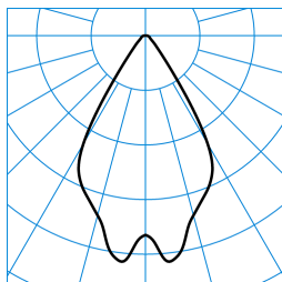
InperlaLP C05 BR22 2700-830 03 + ZN-PC TX041569 ■ C0 - C180
