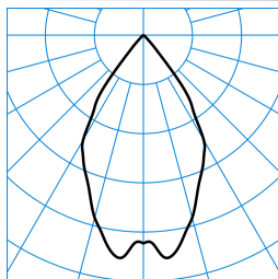
InperlaLP C05 BR22 2700-830 03 TX040952 ■ C0 - C180
