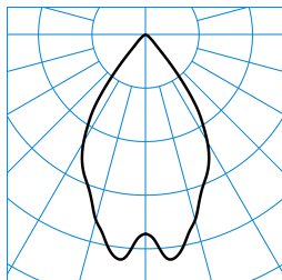
InperlaLP C05 BR22 2700-830 03 + DA 01 TX041563 ■ C0 - C180 ■ C90 - C270
