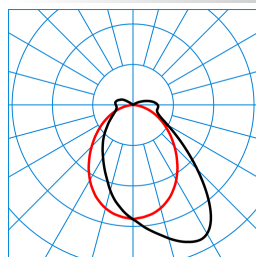
AragFHE 12 PAW 40-940 ET PC TX194616
