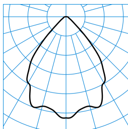
InperlaLP C05 HR22 IP 1800-840 03 + ZN-PC ■ C0 - C180 TX373680
