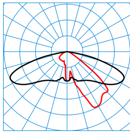
Publisca P1-AB2L-LR/5100-740 6G1S TX047538 ■ C0 - C180 ■ C90 - C270 DIN 5040: A30 UTE: 1,00 G CEN Flux Code: 35 74 97 100 100
