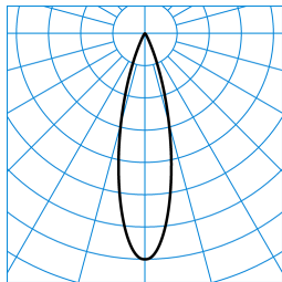
E-Line 7651 LentyP L-MF 30-BC M49 ET 03 (225) TX463260
