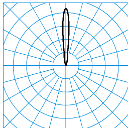
Altigo G2 120 RE1L/4000-830 1G1P + G2 VE IP66 24V DC 240W ■ C0 - C180 TX113669 DIN 5040: E04 UTE: 0,00 J + 0,99 T CEN Flux Code: 0 0 0 0 99 98 99 100 100
