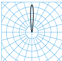
Altigo G2 120 RE1L/4000-830 1G1P + G2 VE IP66 24V DC 120W TX113668
