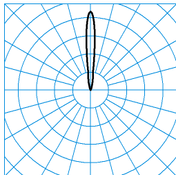
Altigo G2 120 RE1L/4000-830 1G1P + G2 VE IP66 24V DC 30W ■ C0 - C180 TX113670 DIN 5040: E04 UTE: 0,00 J + 0,99 T CEN Flux Code: 0 0 0 0 99 98 99 100 100
