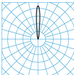
Altigo G2 120 RE1L/4000-830 1G1P + G2 VE IP66 24V DC 80W ■ C0 - C180 TX113671 DIN 5040: E04 UTE: 0,00 J + 0,99 T CEN Flux Code: 0 0 0 0 99 98 99 100 100
