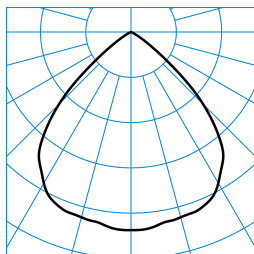
InperiaL G2 C07 BR22 2700-830 01 + DA 01 TX373504 ■ C0 - C180
