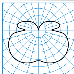
PolaroniQ H2D LED2000-840 ETDD 2,0m TX045259
