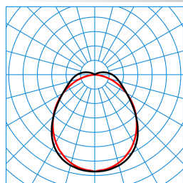
OleveonF 1500 4000-840 PC TX056128
