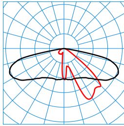
Publisca P1-AB2L-LR/1350-740 2G1S ET (CLO initial value) TX300816 ■ C0 - C180 ■ C90 - C270 DIN 5040: A30 UTE: 1,00 G CEN Flux Code: 34 70 96 100 100
