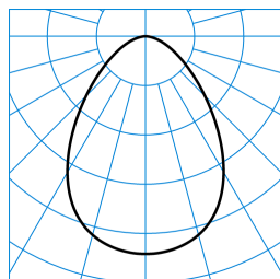
InperlaLP C05 BR25 2700-830 03 + DA-M 03 ■ C0 - C180 TX374535
