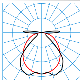
OleveonF 15 B 6000-865 ETDD TX056213
