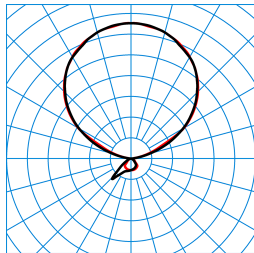
LuceoS S-U PAW-IL 170-830 03(LEO2) TX371992
