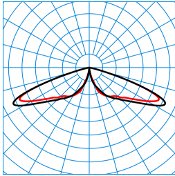
CS 19 100-RB6L-LR/2200-730 2G1S ET (CLO end value) TX300079
