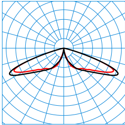
CS 19 100-RB6L-LR/2200-730 2G1S ET (CLO initial value) TX300080
