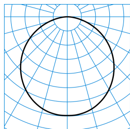
Olisq RWD1 DW 10-840 ETDD IP54 PC + Olisq RWD1 ZDR 1/1 01 TX425640
