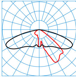
Publisca P1-AB2L-LR/4200-730 6G1S ET (CLO initial value) TX301645 ■ C0 - C180 ■ C90 - C270 DIN 5040: A30 UTE: 1,00 G CEN Flux Code: 35 74 97 100 100
