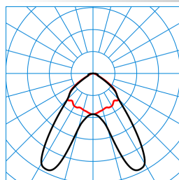
7651 LightP DA-B-DA 80-840ET L75 01 (150) TX557116
