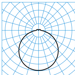
Olisq RWD3 DW 30-840 ETBLE +DMM + Olisq RWD3 ZDR 1/2 03 TX426662
