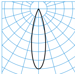
E-Line 7651 LentyP L-MF 40-835 M34 ETBLE 03 (225) TX463434
