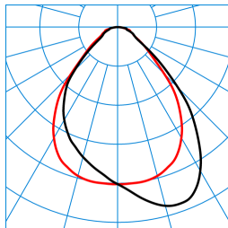
ArimoFit G2 Act M59 P-WW 53-8 ETDD8 (ActDSU) TX376409 ■ C0 - C180 ■ C90 - C270 DIN 5040: A50 UTE: 1,00 C CEN Flux Code: 66 90 97 100 100
