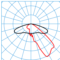
Publisca P1-AB2L-LR/3200-740 4G1S ET (CLO initial value) TX300361 ■ C0 - C180 ■ C90 - C270 DIN 5040: A30 UTE: 1,00 G CEN Flux Code: 35 73 97 100 100
