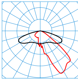
Publisca P1-AB2L-LR/3200-740 4G1S TX047528 ■ C0 - C180 ■ C90 - C270 DIN 5040: A30 UTE: 1,00 G CEN Flux Code: 35 73 97 100 100
