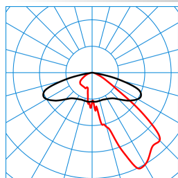
Publisca P2-AB2L-LRA/3500-740 4G1S TX047795 ■ C0 - C180 ■ C90 - C270 DIN 5040: A30 UTE: 1,00 G CEN Flux Code: 35 73 97 100 100
