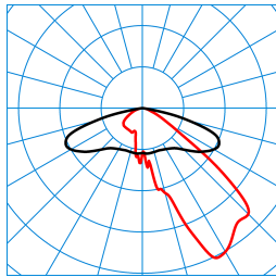
Publisca P1-AB2L-LRA/3500-740 4G1S ET (CLO end value) TX3013591 ■ C0 - C180 ■ C90 - C270 DIN 5040: A30 UTE: 1,00 G CEN Flux Code: 35 73 97 100 100
