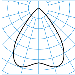
InperiaL G2 C07 BR19 2700-840 03 TX052851 ■ C0 - C180
