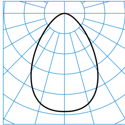
InperiaL G2 C07 BR19 2700-840 03 + DA-M 03 TX052853 ■ C0 - C180 ■ C90 - C270
