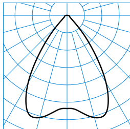
InperiaL G2 C07 BR19 2700-840 03 + ZN-PC TX052856 ■ C0 - C180
