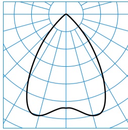
InperiaL G2 C07 BR19 2700-840 03 + RD-PC TX052854 ■ C0 - C180
