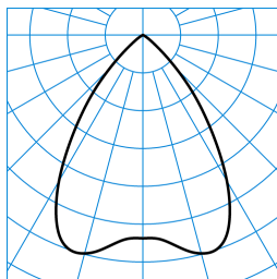
InperiaL G2 C07 BR19 2700-840 03 + DA 03 TX052852 ■ C0 - C180
