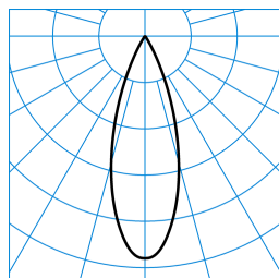
E-Line 7651 Lentyp L-FL 30-840 M35 ET 01 (225) TX463222
