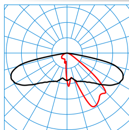
Publisca P1-AB2L-LR/2000-740 3G1S TX047518 ■ C0 - C180 ■ C90 - C270 DIN 5040: A30 UTE: 1,00 l CEN Flux Code: 34 71 96 100 100
