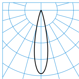
E-Line 7651 LentyP L-SP 30-827 M32 ET 03 (225) TX463598
