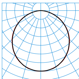
Olisq QWD3 DW 45-830 ET EB3 IP54 IK + Olisq QWD3 ZDR 1/1 01 TX461653
