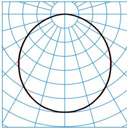
Olisq QWD3 DW 45-830 ET EB3 IP54 IK + Olisq QWD3 ZDR 1/1 03 TX461357
