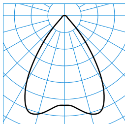
InperiaL G2 C07 HR19 2700-840 01 + ZN-PC ■ C0 - C180 TX373472
