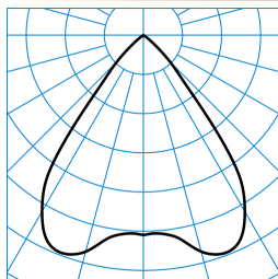
InperiaL G2 C07 HR19 2700-840 01 ■ C0 - C180 TX373477
