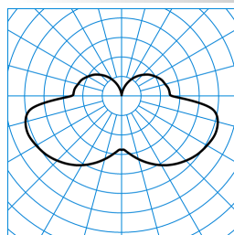
PolaronIQ WD2 LED2000-830 ET TX371779
