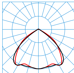
7651 LightP B-B-B 65-830ET L75 03 (225) TX558131
