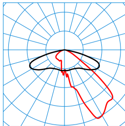
Publisca P1-AB2L-LRA/3200-740 4G1S TX047565 ■ C0 - C180 ■ C90 - C270 DIN 5040: A30 UTE: 1,00 G CEN Flux Code: 35 73 97 100 100
