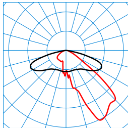
Publisca P1-AB2L-LRA/3200-740 4G1S ET (CLO end value) TX300448 ■ C0 - C180 ■ C90 - C270 DIN 5040: A30 UTE: 1,00 G CEN Flux Code: 35 73 97 100 100
