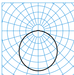
Olisq RWD4 DW 40-840 ETBLE +DMM IP54 + Olisq RWD4 C 01 TX427048
