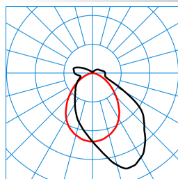
TugraHE Act 18 PAW 70-840 ETDD8 01 (ACTDWW) TX303304 ■ C0 - C180 ■ C90 - C270 DIN 5040: B40 UTE: 0,87 E + 0,13 T CEN Flux Code: 48 79 93 87 100 7 25 60 13
