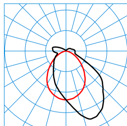
TugraHE Act 18 PAW 70-840 ETDD8 01 (ACTDSU) TX302573 ■ C0 - C180 ■ C90 - C270 DIN 5040: B40 UTE: 0,87 E + 0,13 T CEN Flux Code: 48 79 93 87 100 7 25 60 13
