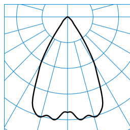
InperlaLP C05 HR22 2700-840 01 + RD-PC ■ C0 - C180 TX373674
