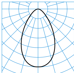
InperiaLP C05 HR22 2700-840 01 + DA-M 01 TX373676 ■ C0 - C180
