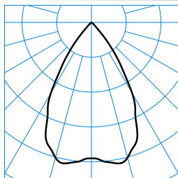
InperiaLP C05 HR22 2700-840 01 TX373677 ■ C0 - C180
