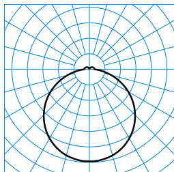
Olisq RWD2 DW 40-830 ETBLE +DMR IP54 PC + Olisq RWD2 ZDR 1/2 01 TX426097
