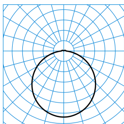
Olisq RWD2 DW 40-830 ETBLE +DMR IP54 PC + Olisq RWD2 C 01 TX425825
